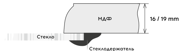
Фасад без выборки под стекло
