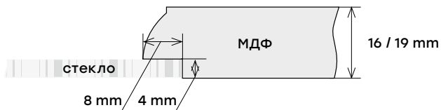
Фасад с выборкой под стекло МДФ 16, 19 мм
