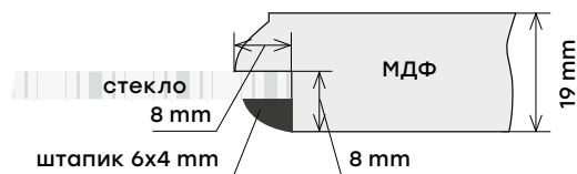
Фасад с выборкой под стекло МДФ 19 мм
